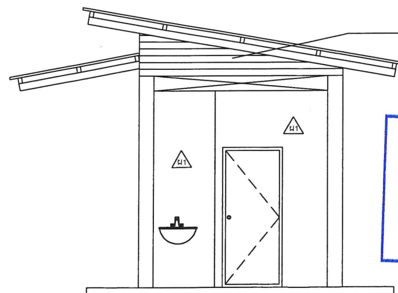
รูปด้านขวา scale 1:50
