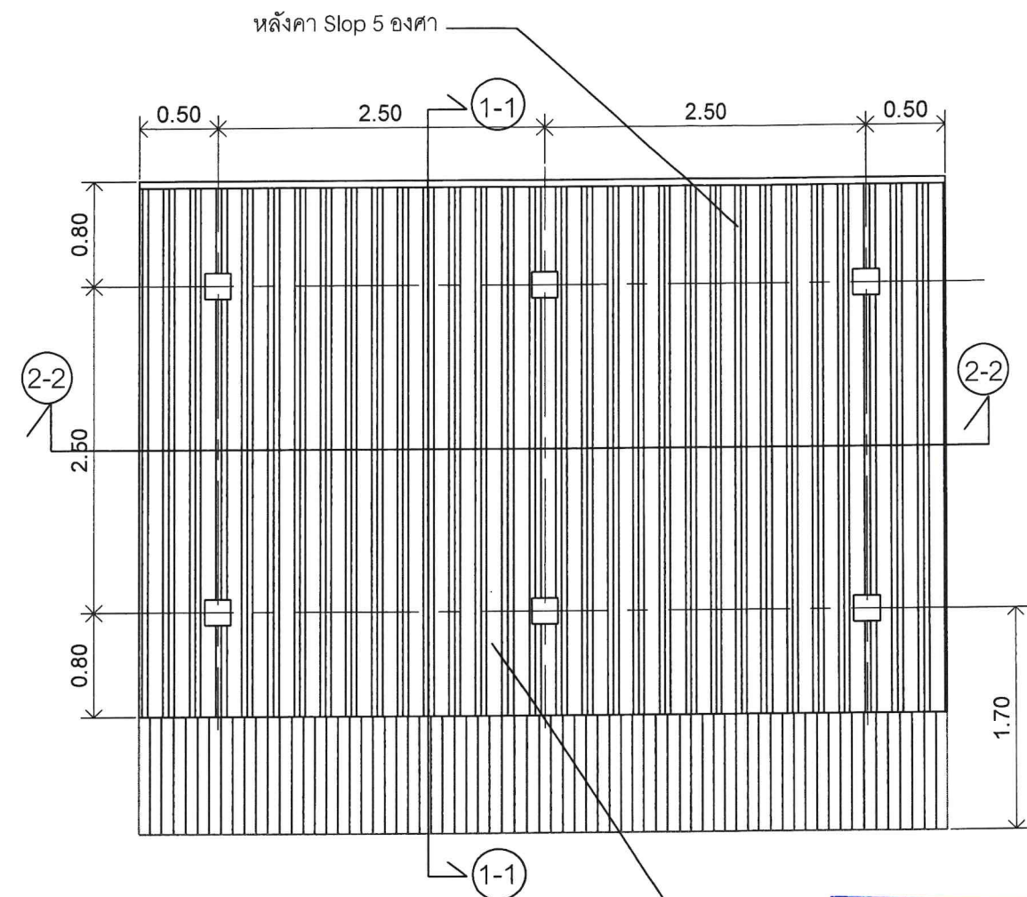
แปลนหลังคาห้องน้ำ Scale 1:50
