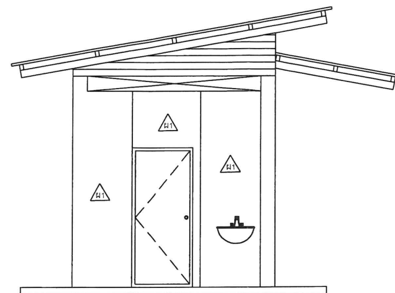
รูปด้านซ้าย scale 1:50
